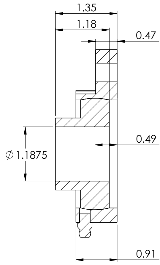
SECTION A-A SCALE 4 : 5
